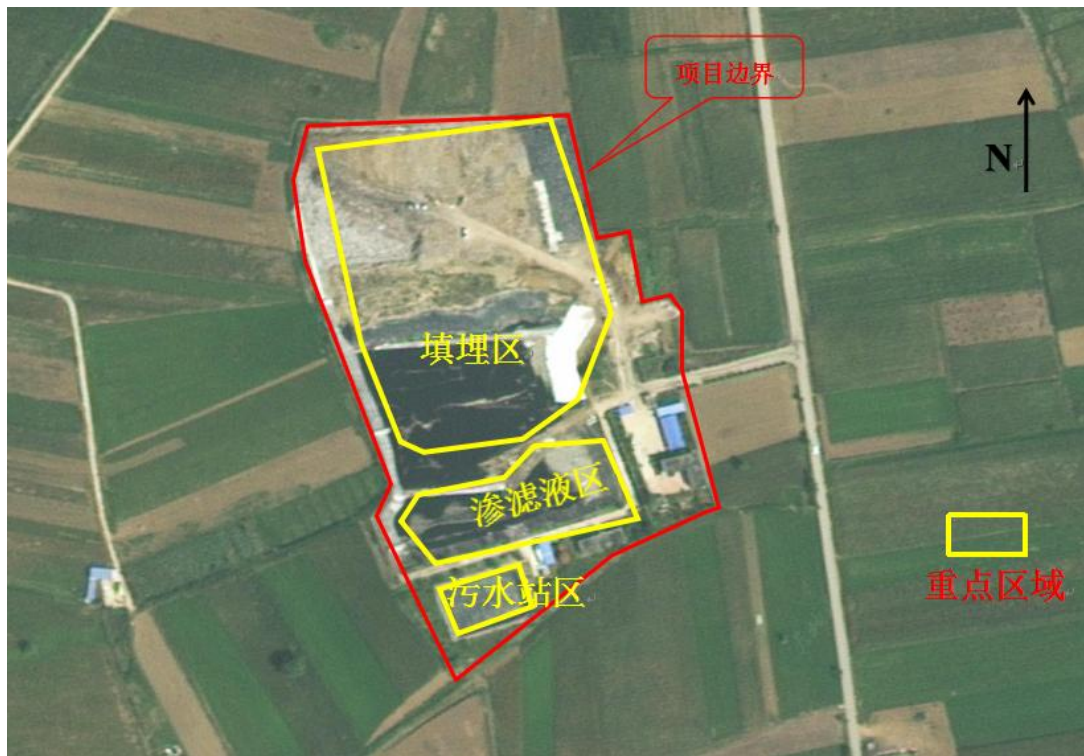
图4-2项目平面布置图
